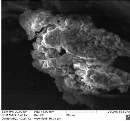
Рисунок 12. Хлорид серебра
