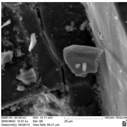
Рисунок 7. Железо-титановые микрочастицы
